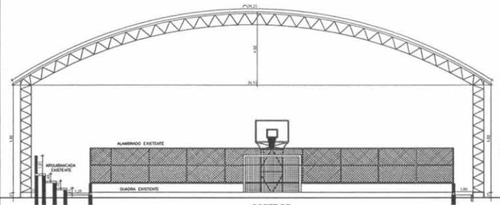
CORTE BB ESC. 1/100
