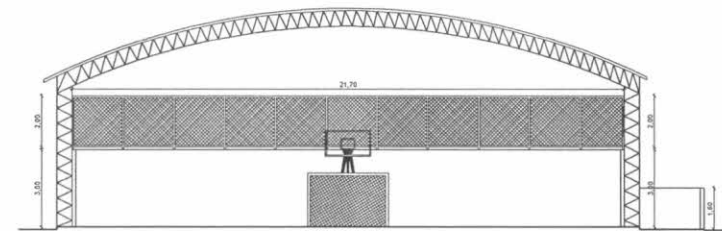
CORTE BB ESC. 1:100
