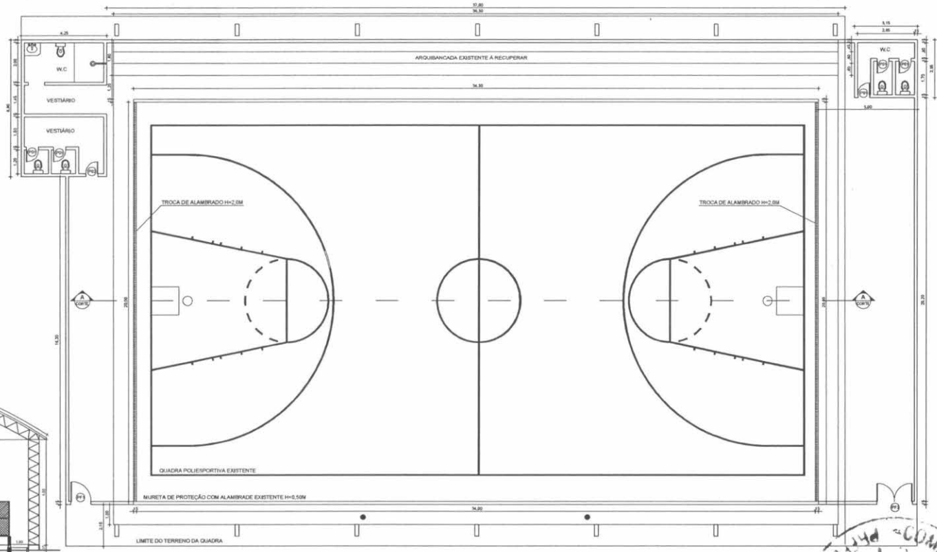
PLANTA BAIXA ESC. 1/100
