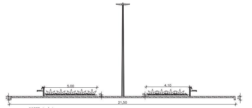
CORTE A / A ESC.: ..... 1/75
